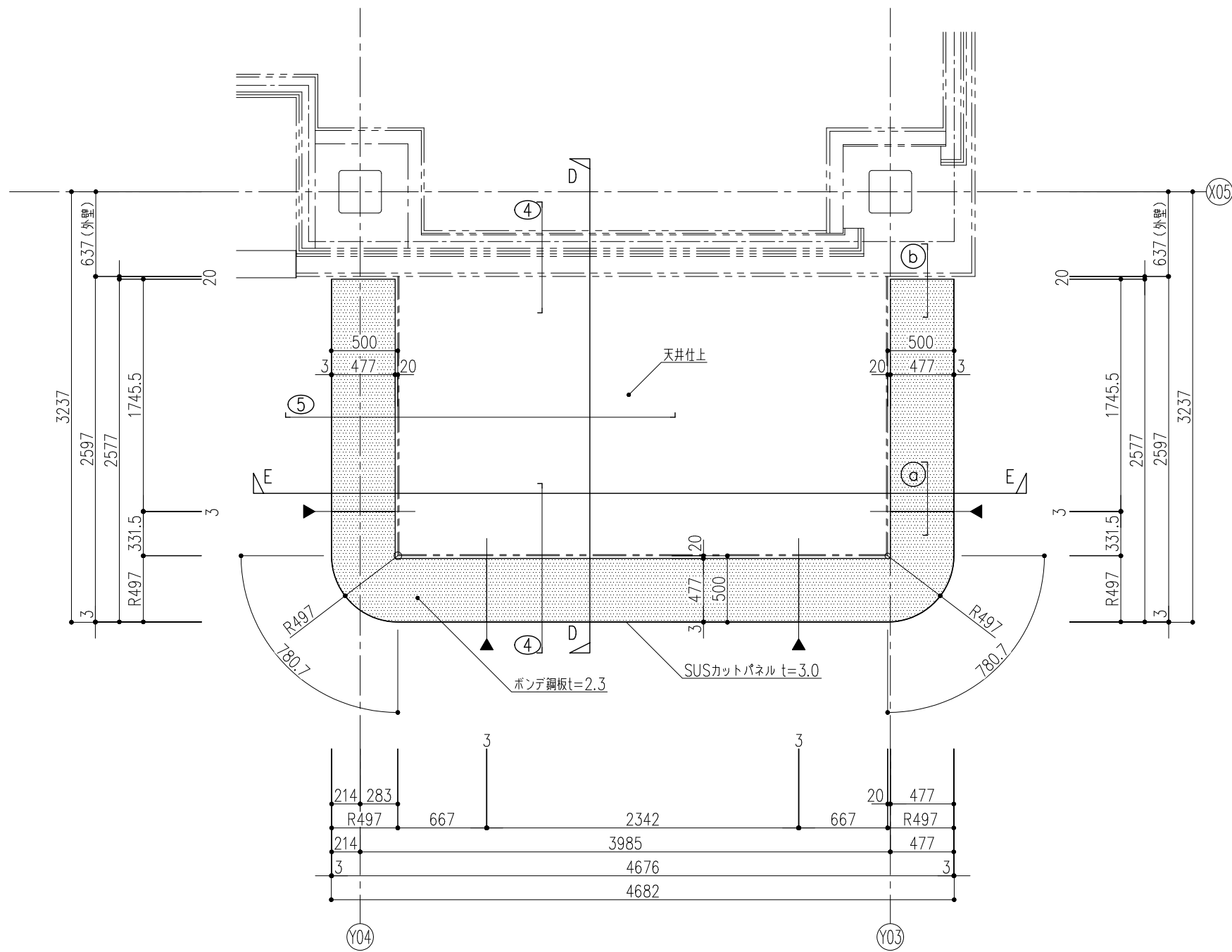
2F ボンデ鋼板平面図
