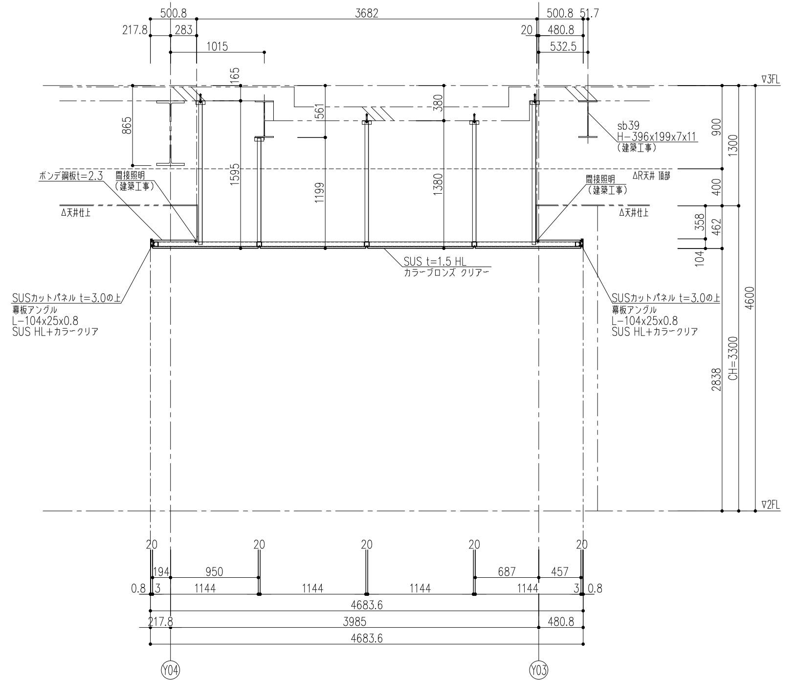
E断面図
