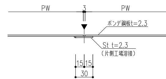
a部詳細図 (1/2)
