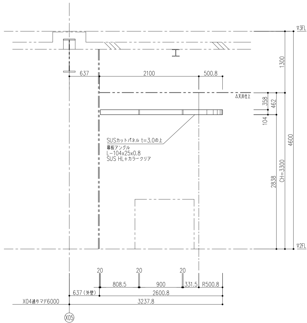
B立面図
