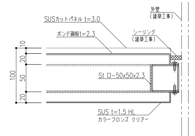
b部詳細図 (1/2)
