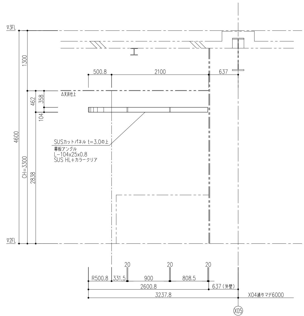
C立面図
