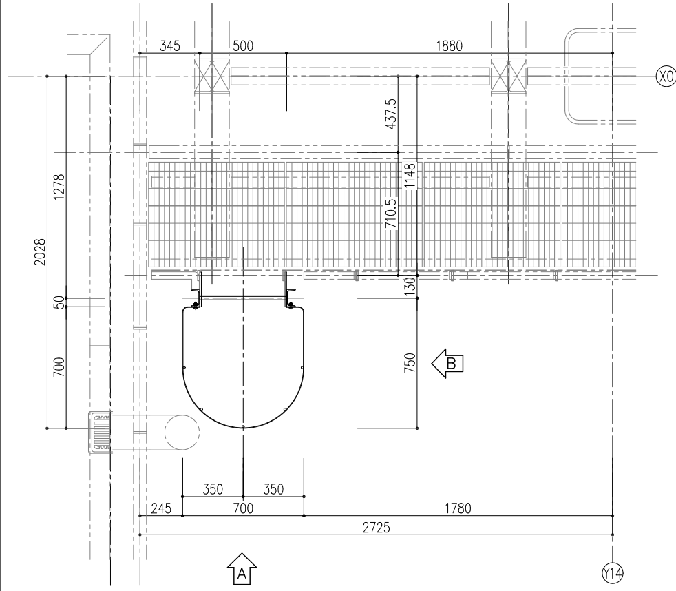
平面図
