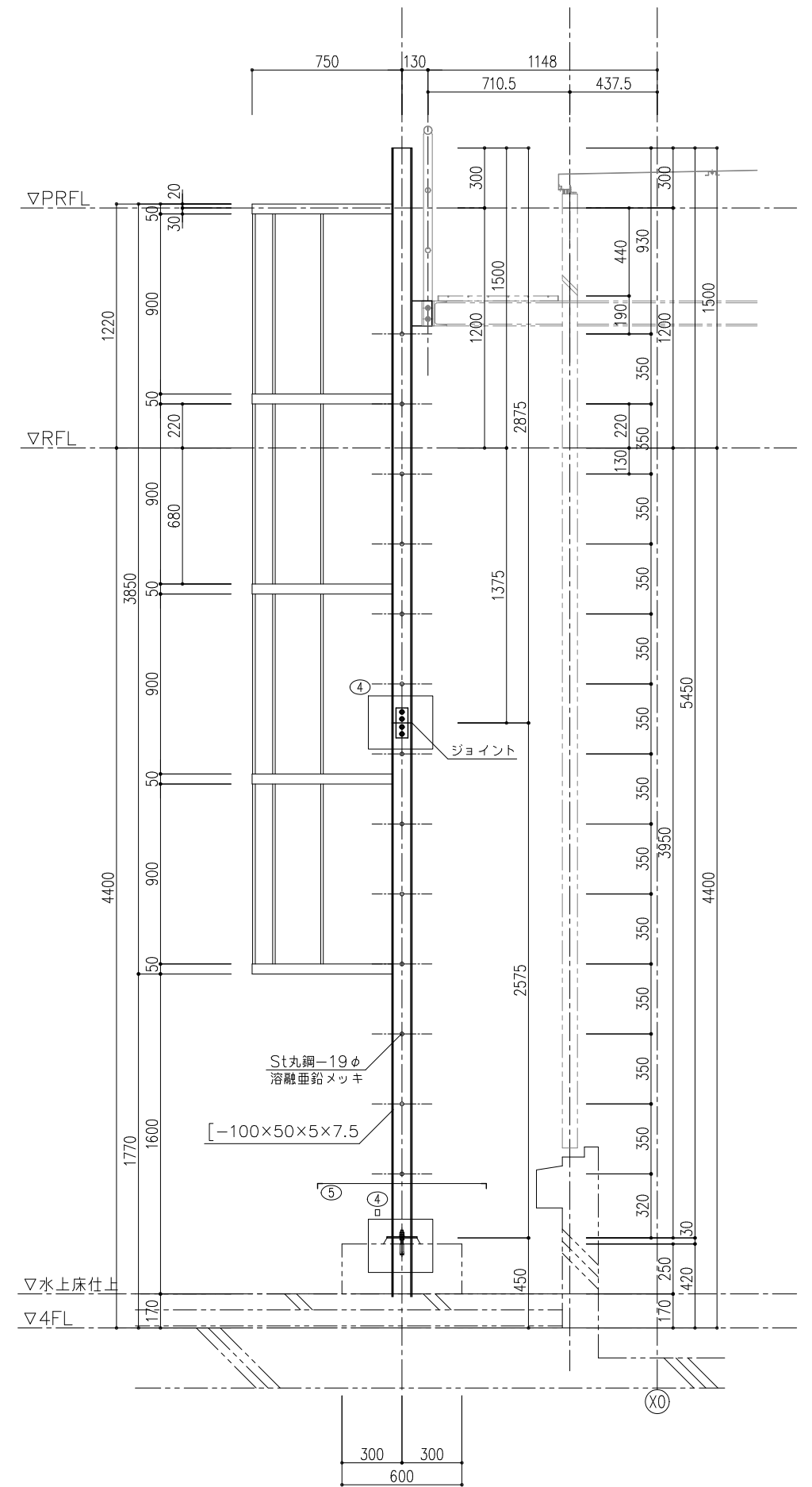
B立面図
