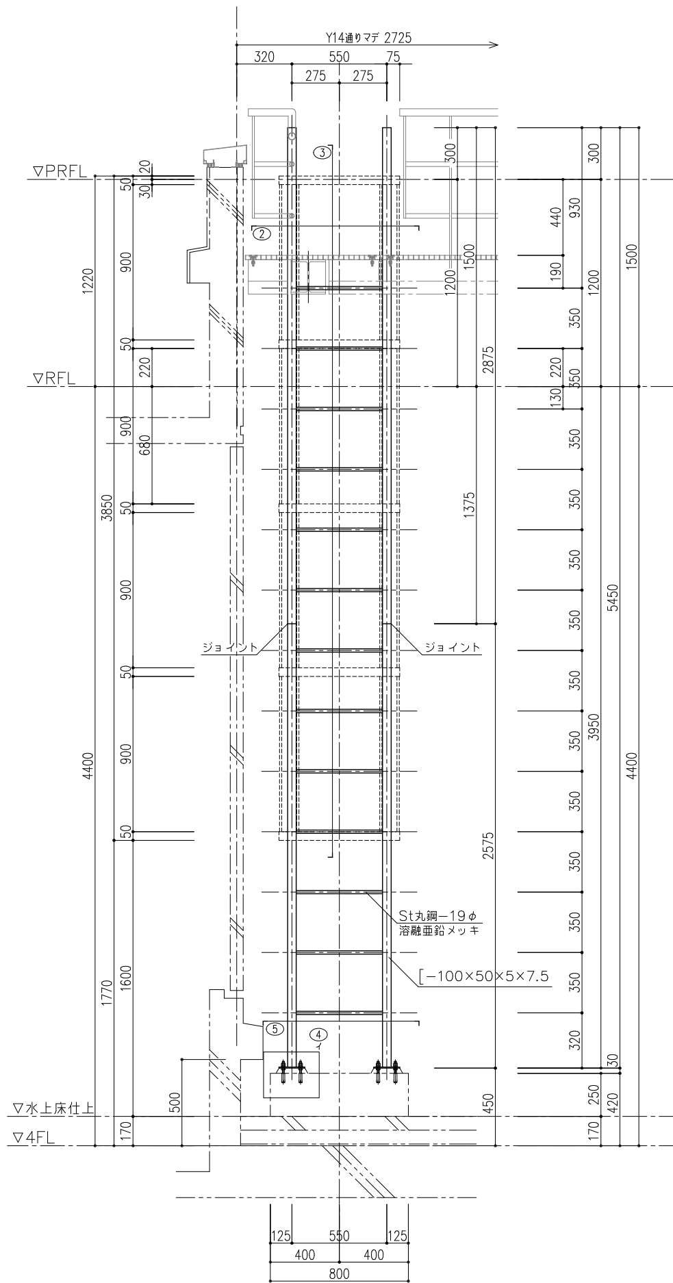
A立面図
