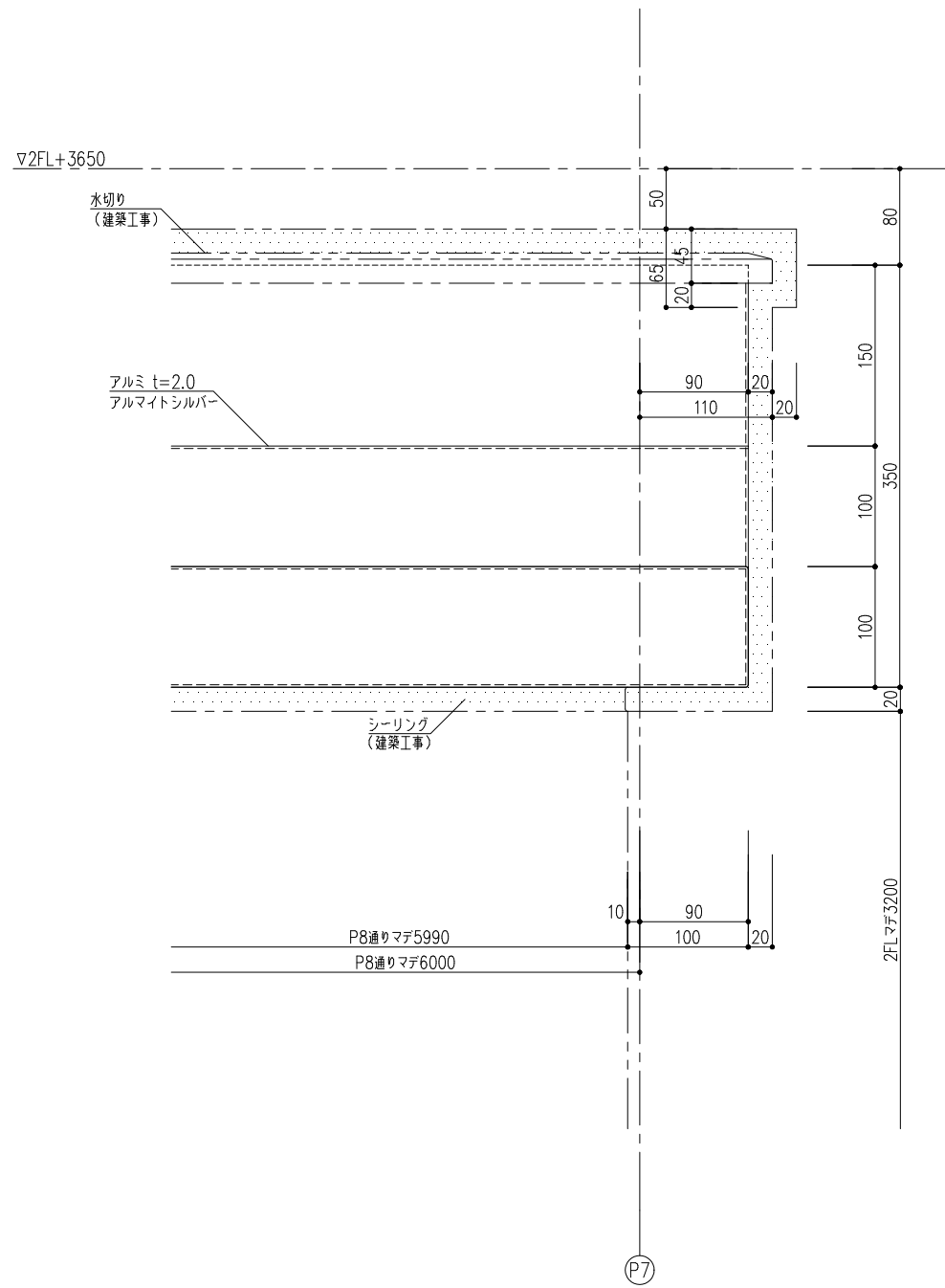
拡大立面図
