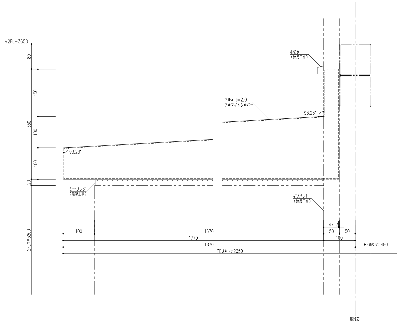
拡大立面図
