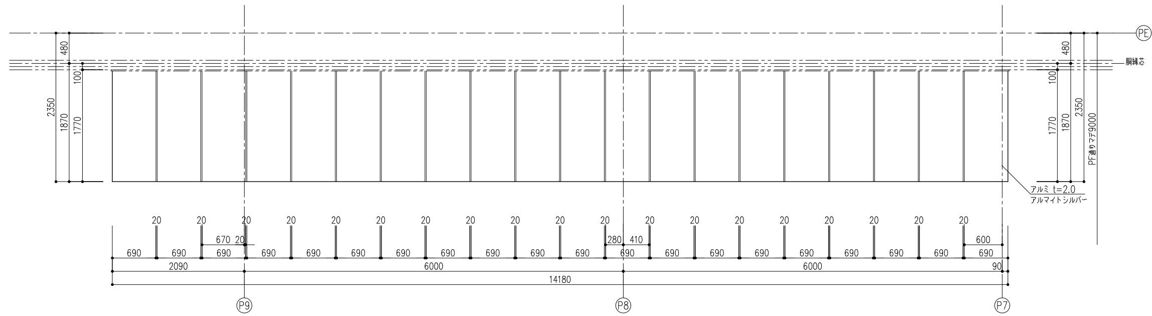
平面図
