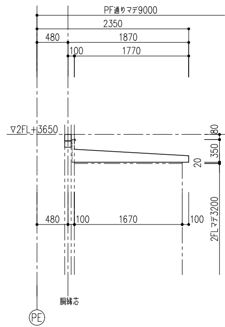
立面図
