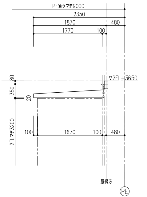
立面図
