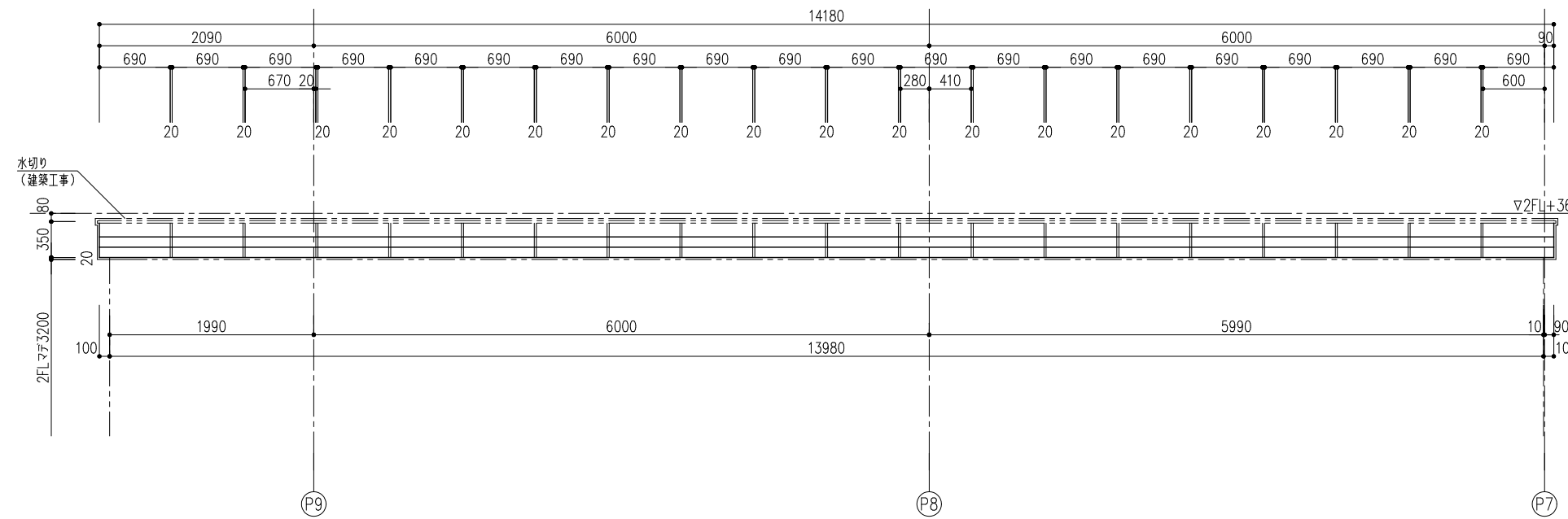
立面図
