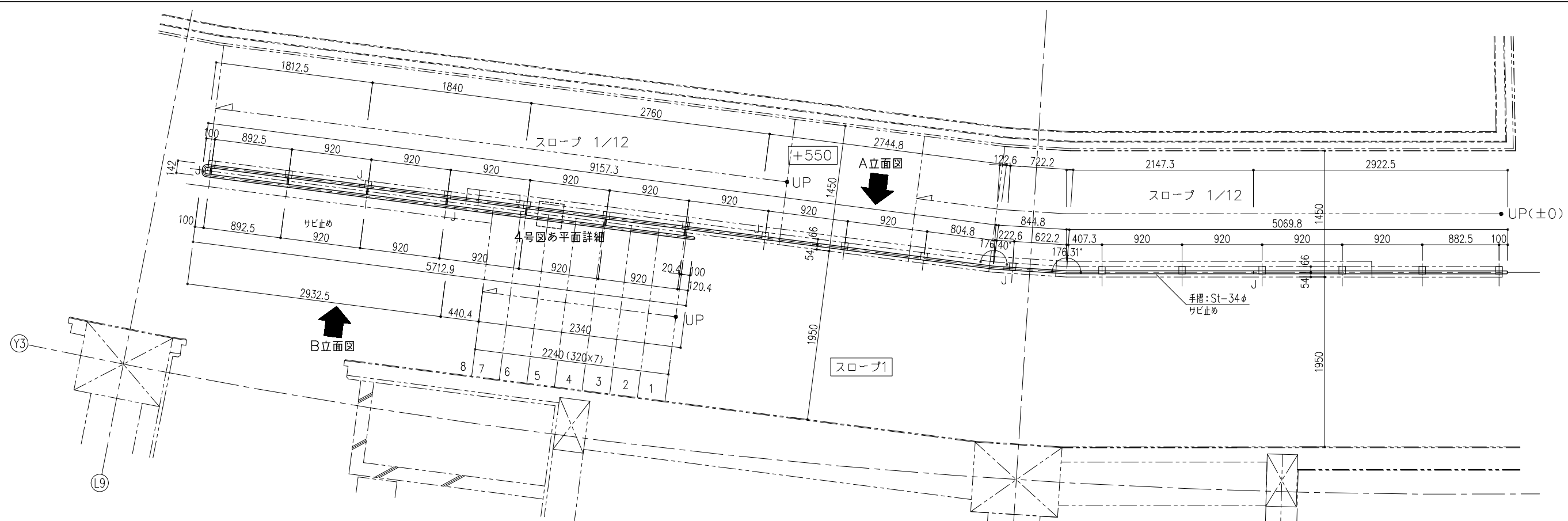
イ部 平面図 (Aタイプ手摺)
