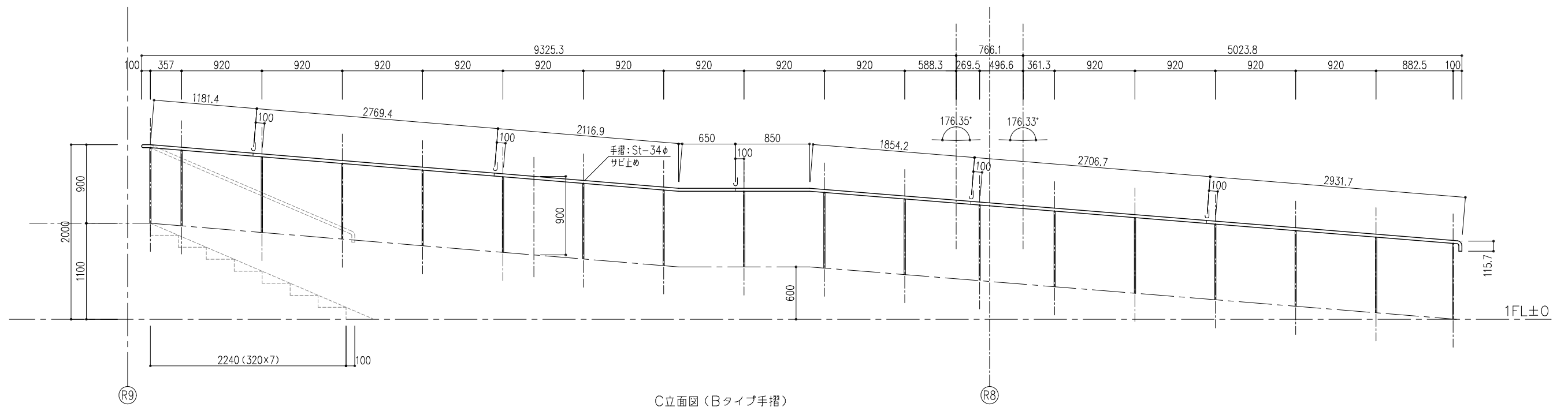
C立面図 (Bタイプ手摺) 詳細7・8号図参照
