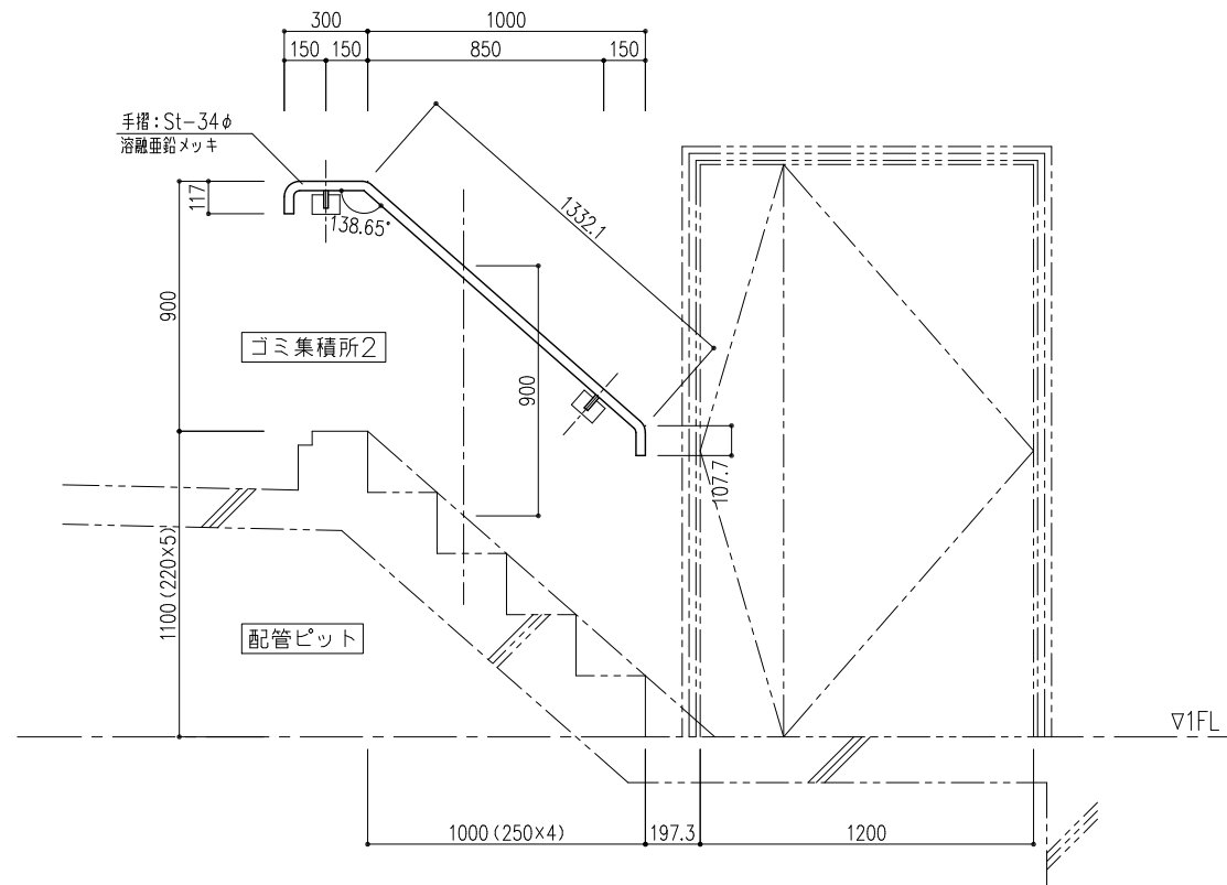
E立面図 (Aタイプ手摺) 詳細6号図参照
