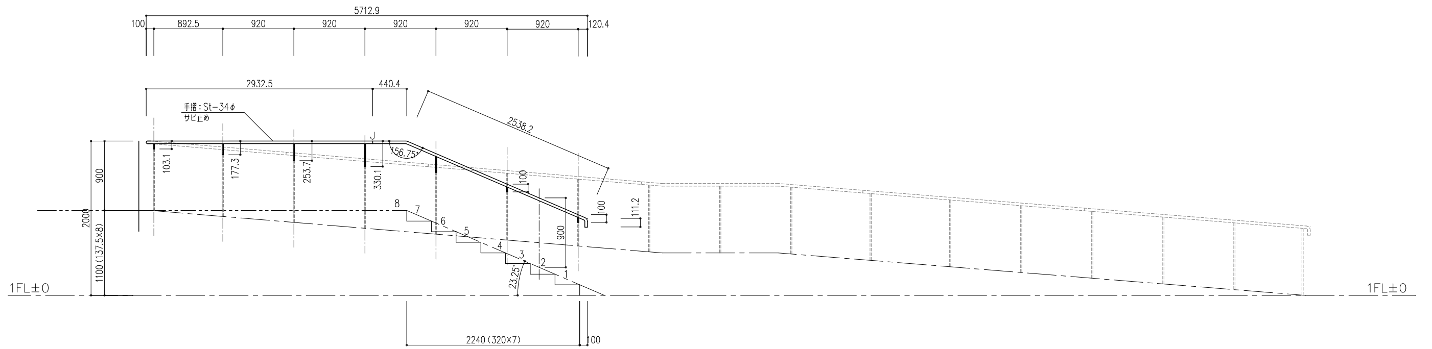
B立面図 (Bタイプ手摺)
