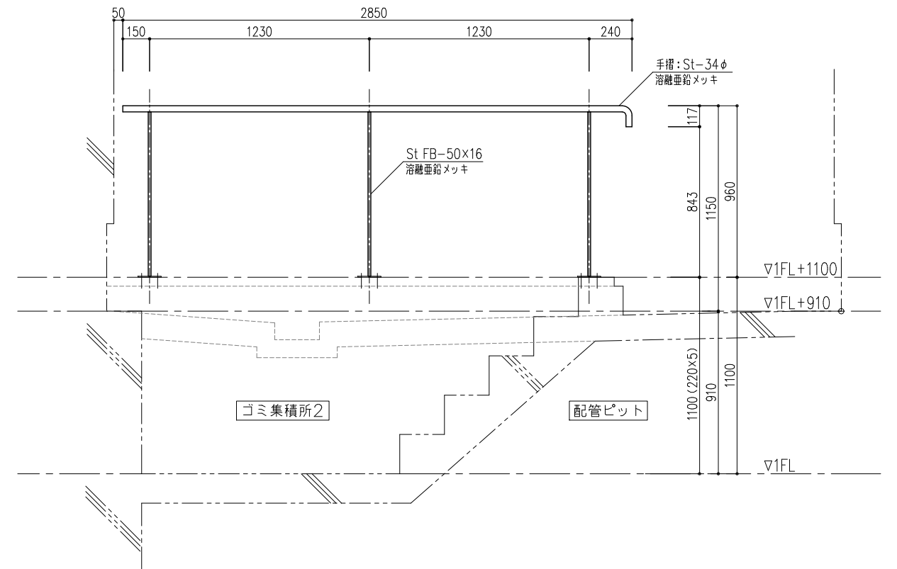
F立面図 (Bタイプ手摺) 詳細9号図参照
