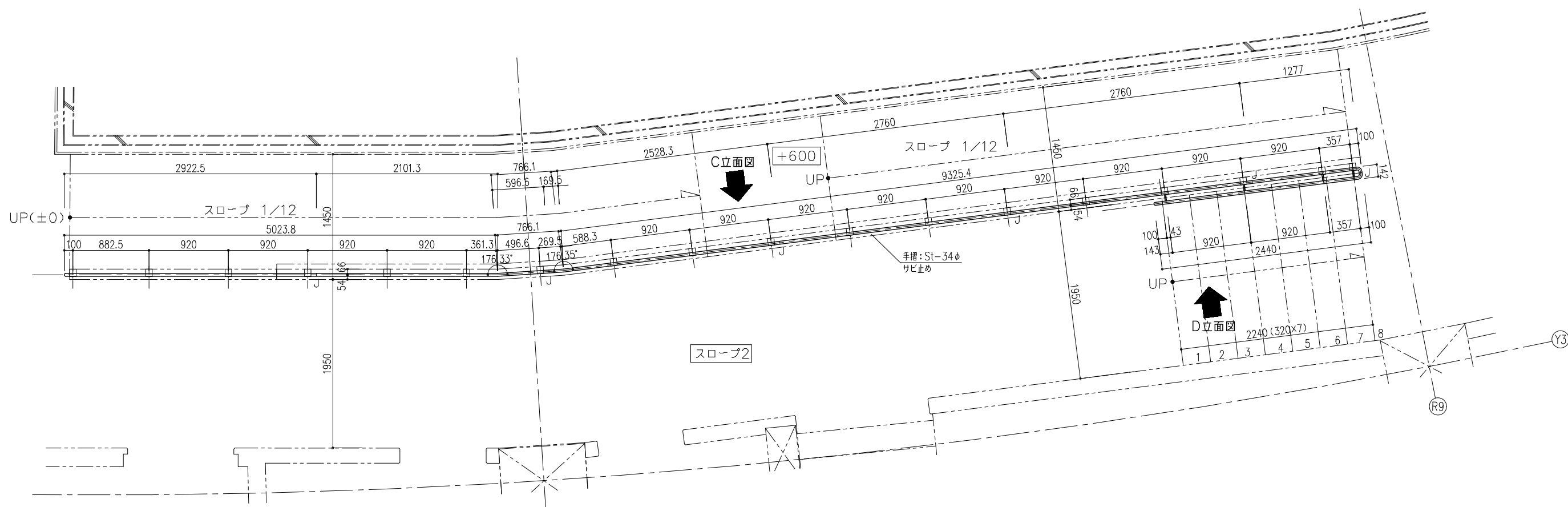
ロ部 平面図 (Aタイプ手摺)
