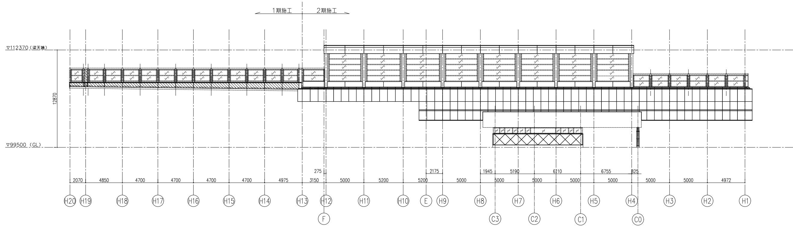
西面立面图
