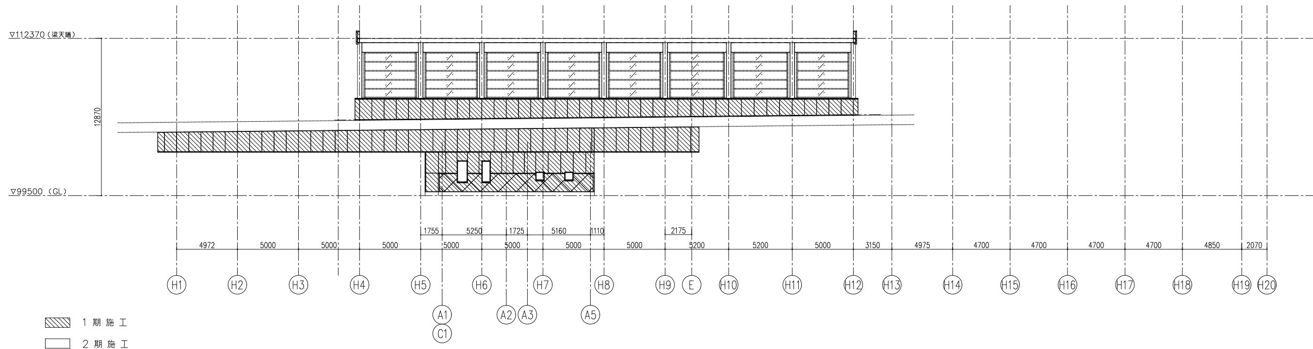
东面立面图 1期施工
